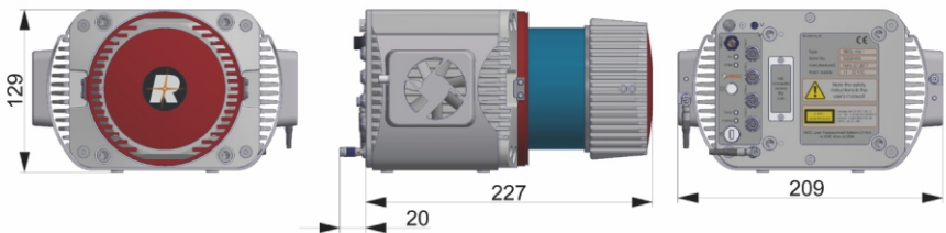
前视图
