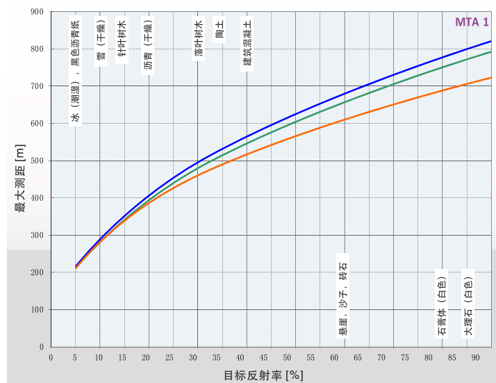
激光脉冲重复频率 100 kHz
