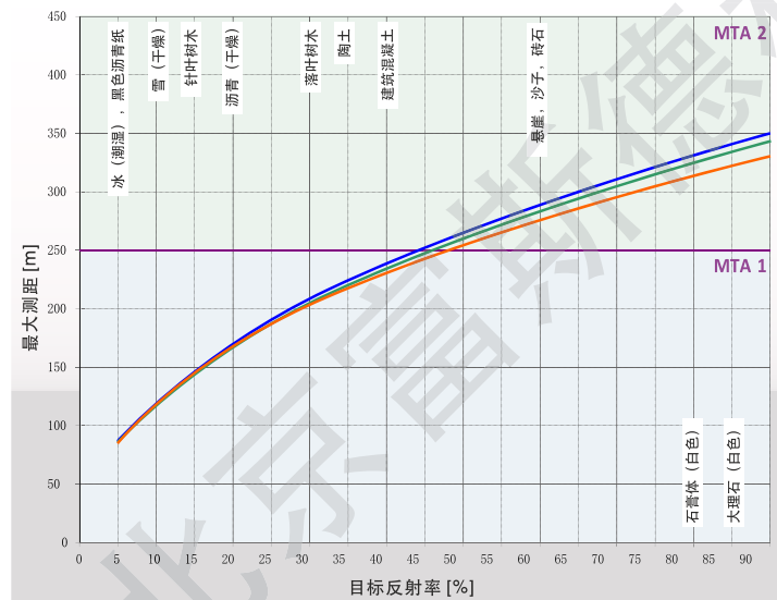
激光脉冲重复频率 600 kHz
