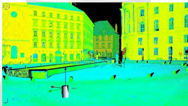
点云假彩色显示 (与距离无关的反射率模式)
